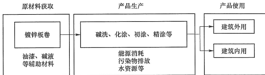
图 B.1 建筑用高强高耐蚀彩涂板生命周期系统边界示意图
